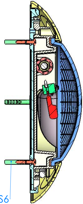
SECCIÓN A-A
