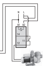
FILTER PUMP Control de filtración 7 y 8
