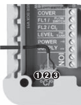
Sonda temperatura 1 rojo 2 amarillo 3 negro
