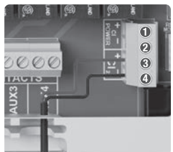
Sonde Vrij Chloor ③ rood ④ zwart
