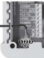
Temperatursonde 1 rot 2 gelb 3 schwarz
