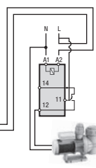
FILTER POMP Controle filtratien ⑦ en ⑧
