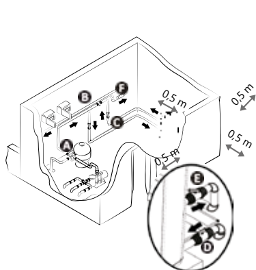
Beltéri telepítés*
