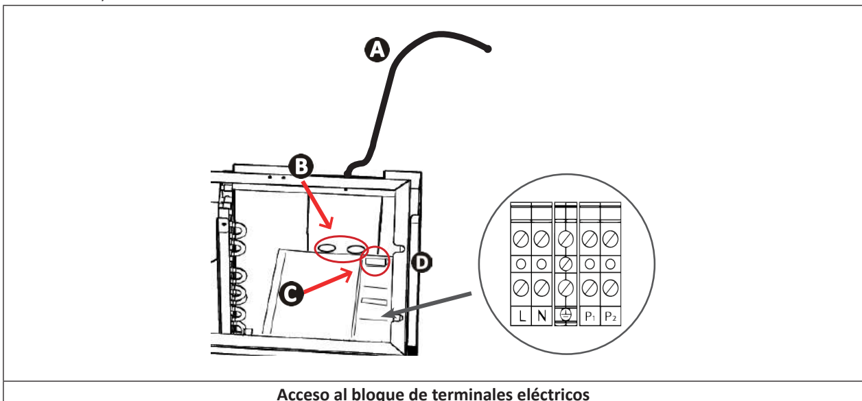
Acceso al bloque de terminales eléctricos
