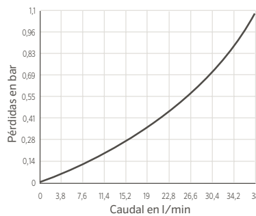
PÉRDIDA DE CARGA EN LOS CODOS ARTICULADOS
