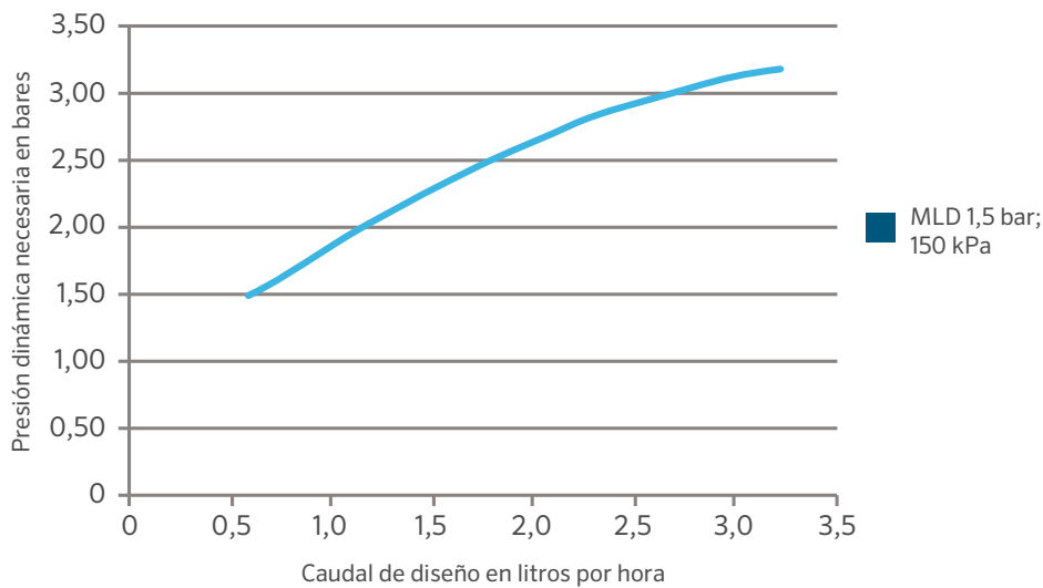
GRÁFICA DEL MLD
