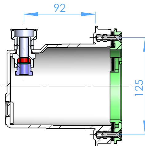
SECCIÓN A-A
