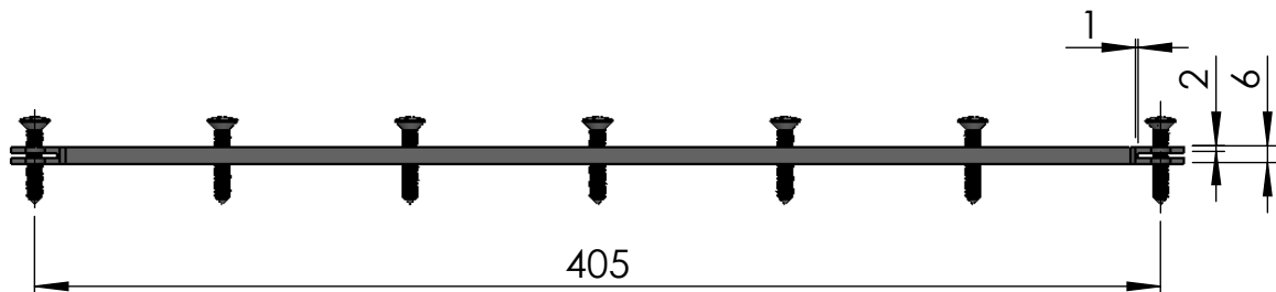
SECCIÓN B-B
